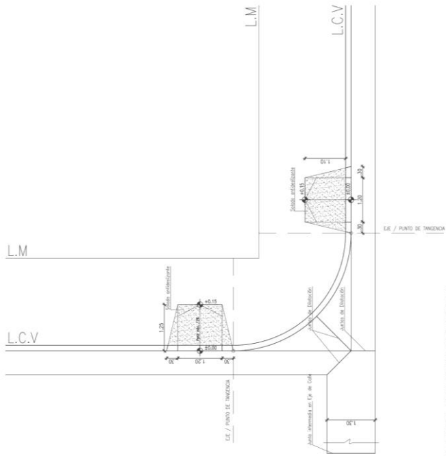
PERFIL RAMPAS DISCAPACITADOS
